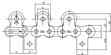
Outer Link Top Roller Installation 외판링크 톱로울러 부착시
