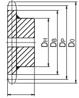
Hub Detachable Type 보드분리형
