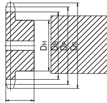
One-side hub extension 한쪽 보스형
